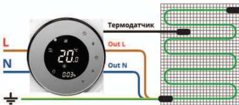
Мал. 3. Схема підключення нагрівального мата ThermoGreen™
